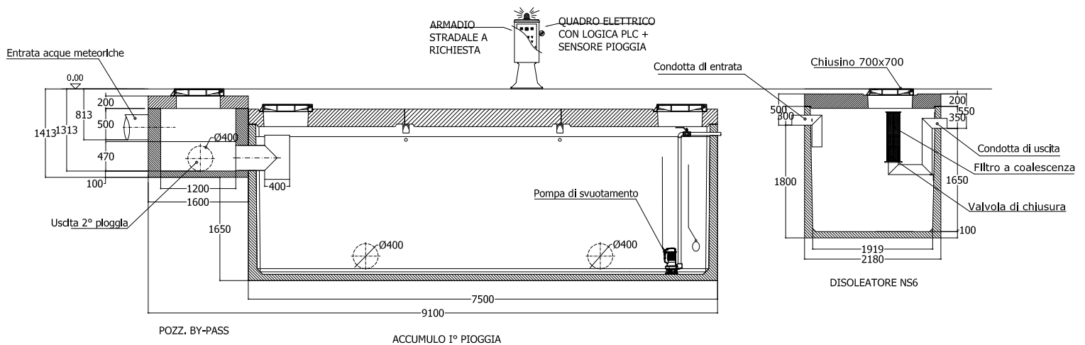
SEZIONE A-A'
