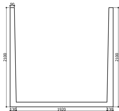
SEZIONE
