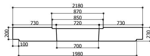
SOLETTA CARRABILE
