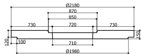
SOLETTA PEDONALE
